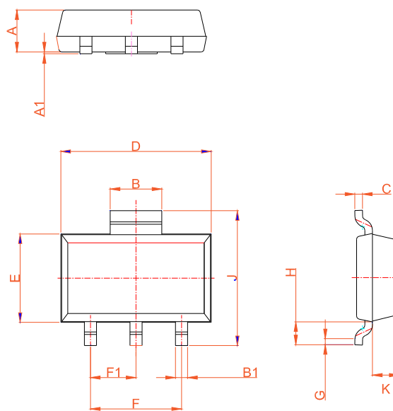
SOT-89
